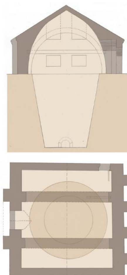
Planta y sección del pozo de nieve
