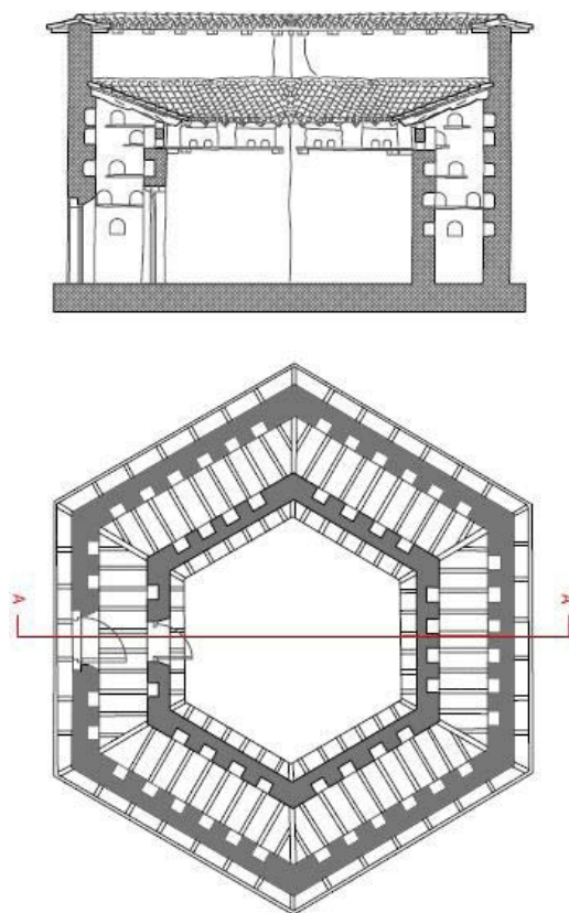
Sección y planta del palomar
