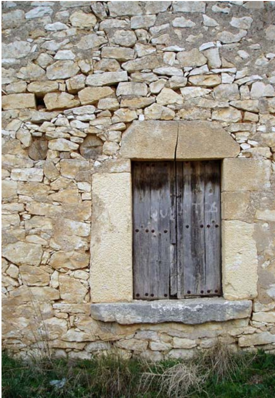
Detalle del hueco de carga de un lagar. Fábrica de mampostería ordinaria y grandes sillares que conforman el hueco
