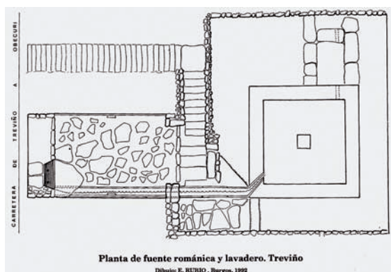
Plano de conjunto de la fuente y lavadero de Treviño
