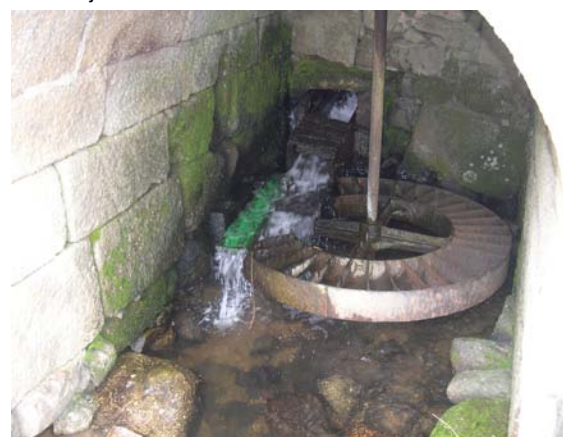
Maquinaria del molino de la Máquina de Fuego, en Villar de la Corneja
